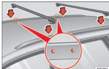
Fig. 185 Leon ST : points de fixation des barres longitudinales pour la galerie porte-bagages du toit.
