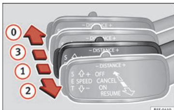
Fig. 204 À gauche de la colonne de direction : troisième levier pour utiliser le régulateur de vitesse adaptatif.
