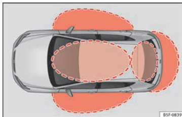
Fig. 132 Système de fermeture et de démarrage sans clé Keyless Access : Zones de proximité.
