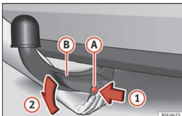
Fig. 242 Libérer la boule amovible
